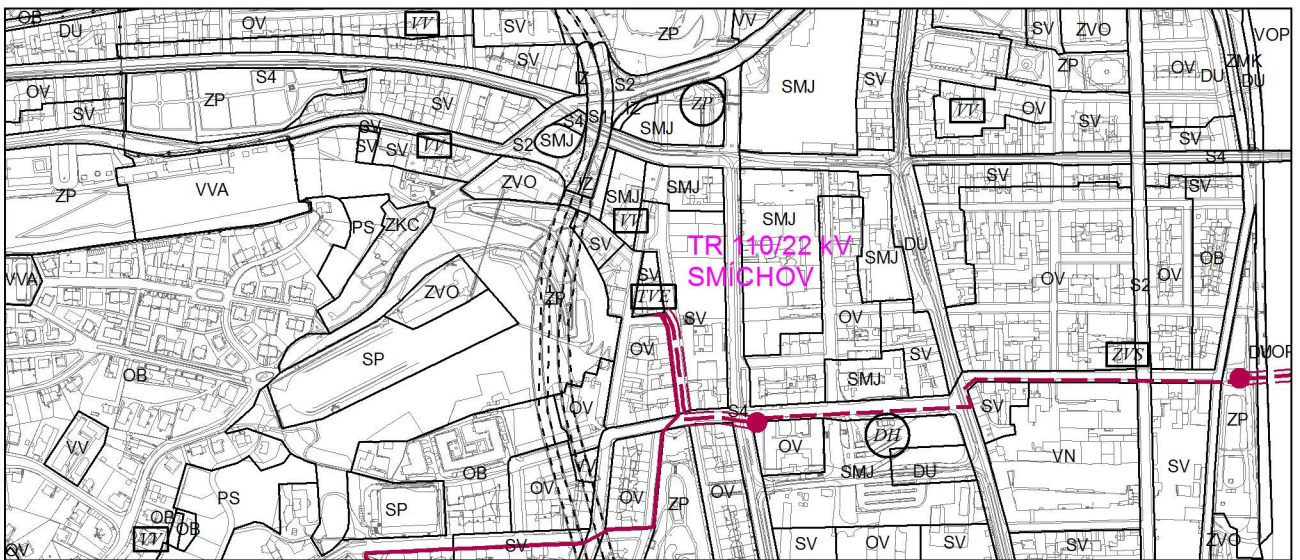
Promítnutí změny do výkresu č. 10 - Energetika
